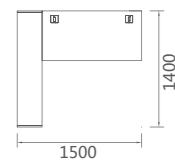
66BG1508 职员位 1500Wx1400Dx1200H (1500)
