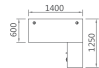
18B1407L 职员位 1400Wx1250Dx760H (1440) 18B1407R 职员位 1400Wx1250Dx760H (1440)
