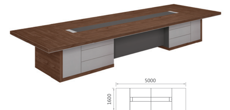
66P5001 会议台 5000Wx1600Dx760H (8420) 66P3601 会议台 3600Wx1400Dx760H (6070)
