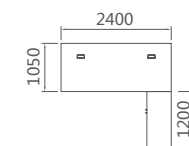
18D2401 大班台 2400Wx1050Dx760H (5333) 18D2001 中班台 2000Wx1050Dx760H (5000)
