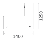
66B1408 职员台 1400Wx1250Dx750H (1440) 副柜可左右互换
