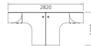
18L2023 屏风位 2820Wx1620Dx1200H (5893)
