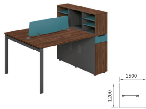
66B1504 职员位 1500Wx1200Dx750H (2280) 66B1304 职员位 1300Wx1200Dx750H (2247)
