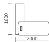
16D2201 主管位 2200Wx1800Dx750H (3010) 16D2001 主管位 2000Wx1800Dx750H (2913)
