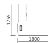
16D1802 主管位 1800Wx1765Dx750H (2470) 16D1602 主管位 1600Wx1740Dx750H (2407)
