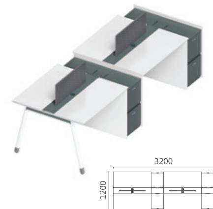
09B3206 职员位 3200Wx1200Dx750H (4517)
